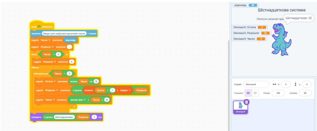
Рисунок 2 — Код програми та результат для числа 46
